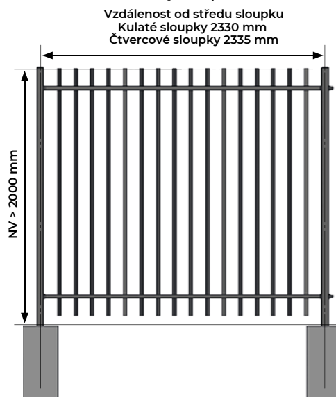
Nominální výška oplocení > 2 m
