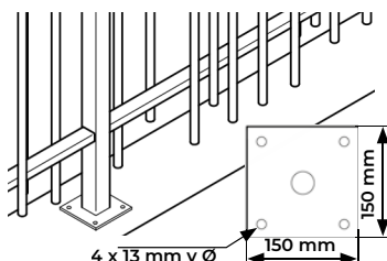
Na základové desce
