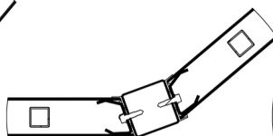
Maximální úhel 140°
