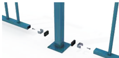
Čtvercové sloupky
